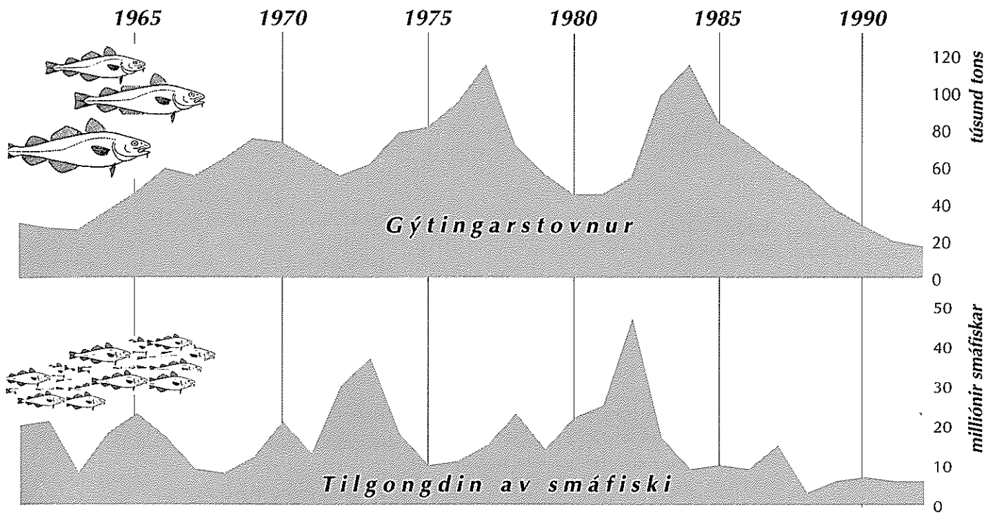
Mynd 1 Ovara farstrikan vísir gýtingarstovnin (í túsund tons) 1961-1992. Síðani 1984 er stovnurin støðugt minkaður. Niðara farstrikan vísir tilgongdina av smáfiski (í mió.) í sama tíðarskeiði.
