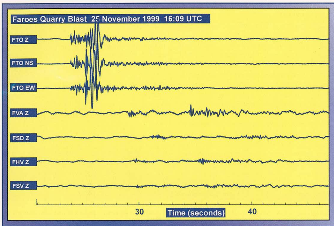
5. mynd: Málðar restingar frá dynamittspreiðing nærhendis Tórshavn.
