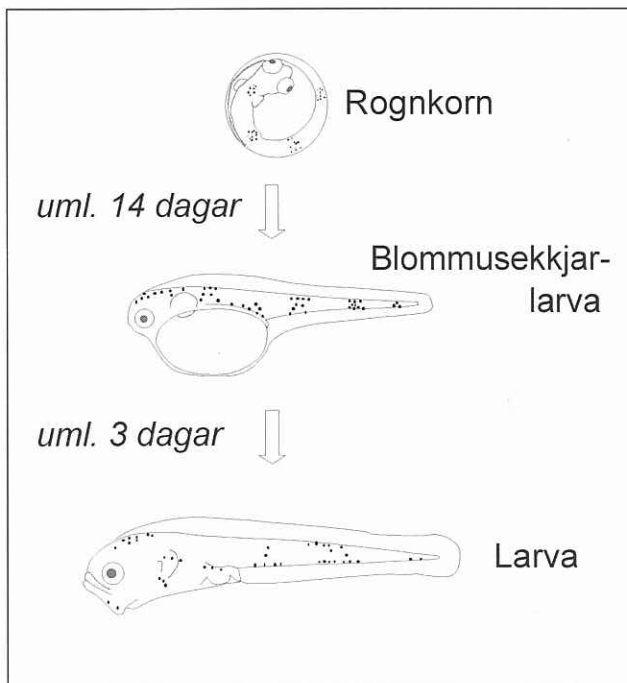
3. mynd Búning frá rognkorni til toskalarvu.
