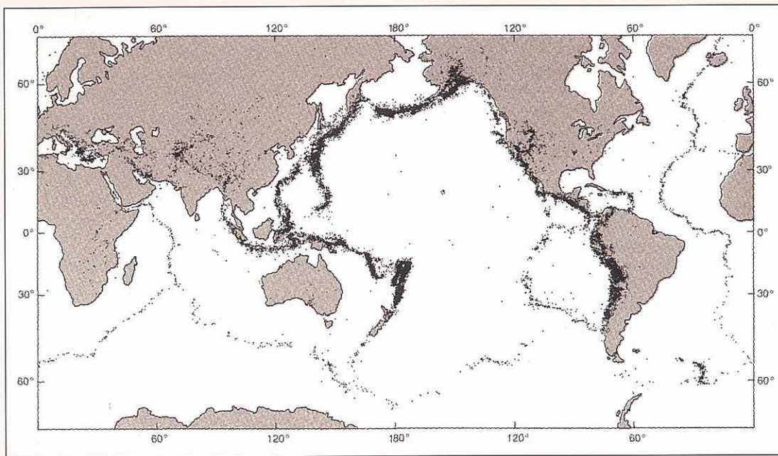
2. mynd. Jarðskjálvtar um heimin. (Heimild: "Earth". Press and Siever, 1974)
