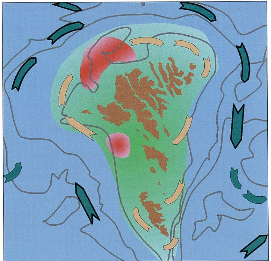
1. mynd Týðningarmestu gýtingarøkini hjá toski á landgrunnum í 1997, 1998 og 1999 (reyð øki). Landgrunssjógvurin (grøna økið) er skildur frá opna havinum (bláa økið). Pílmir vísa nettorákið á landgrunnum, tá ið sjóvarfalsstreymurin er undantikin.
